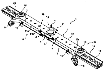
シート装脱着装置の全体図
