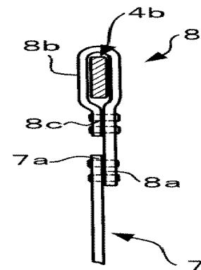
取付け手段の一例を示した概略説明図
