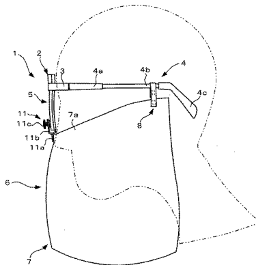
使用状態を側面から示した概略説明図
