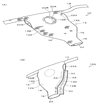
本発明のパウチカバーを示す外観斜視図であり、(A)は実施例 1 を示す図、(B)は実施例 2 を示す図
