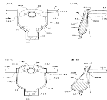
前記実施例 1 と比較例のパウチカバーの使用時の様子を示す正面図及び側面図
