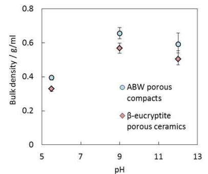
図 ABW成形体とユークリプタイト 多孔体の高密度
