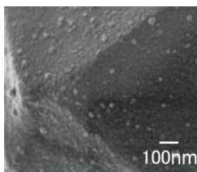
SEMによる表面観察像
